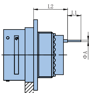
JY27497插座
