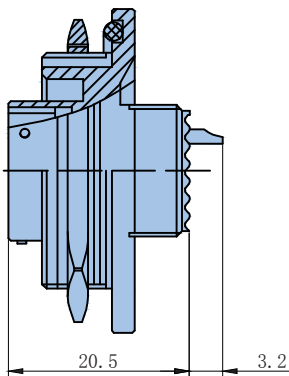
JY27474插座
