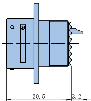
JY27508插座
