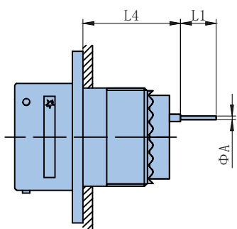
JY27472插座
