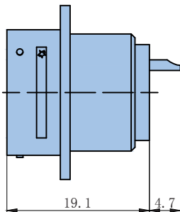
JY27513插座
