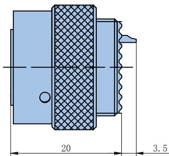
JY27497插座
