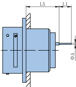
JY27513插座
