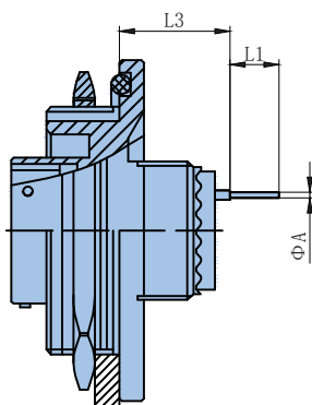
JY27474插座
