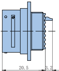
JY27497插座
