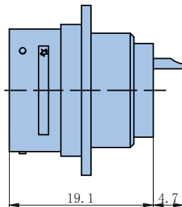
JY27508插座
