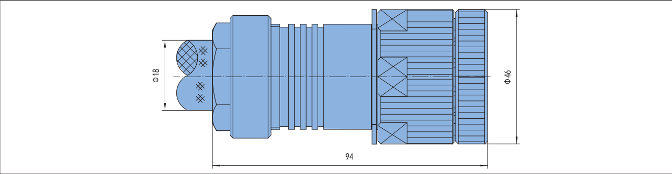
插座 SM42GZ13Z-S-01
