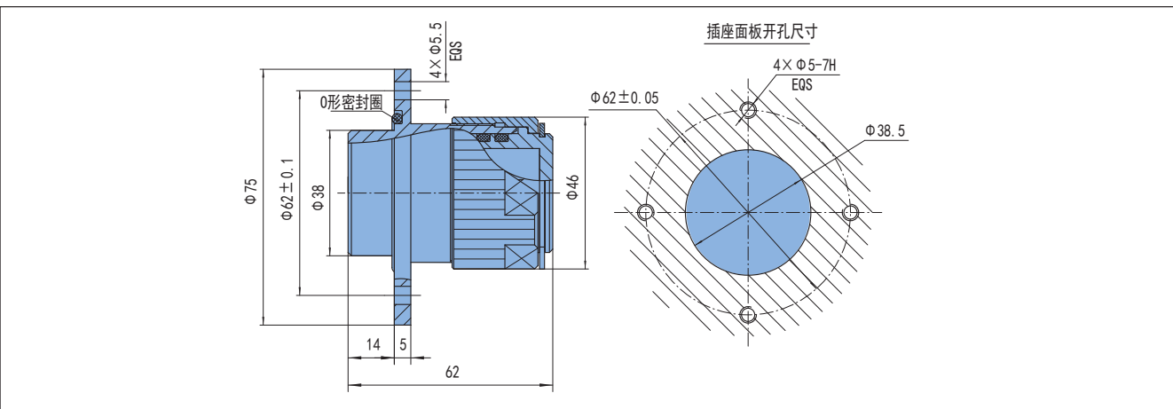
插座 SM42GZ13Z-S-01
