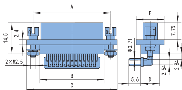
插座J29D-9~37ZKWR7
