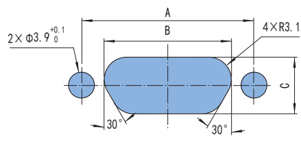
板后安装开孔尺寸：
