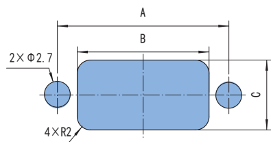
板前安装开孔尺寸：
