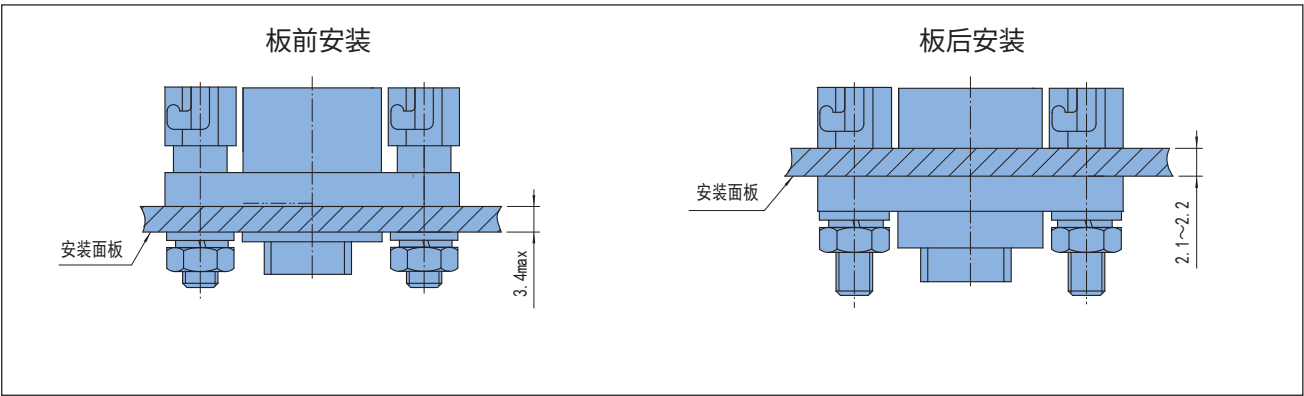
安装示意图
