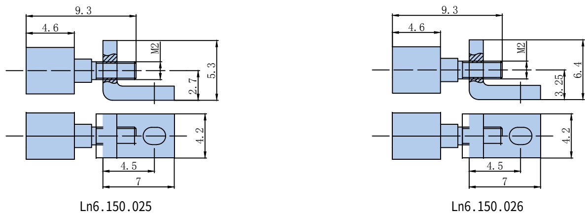
产品外形尺寸图
