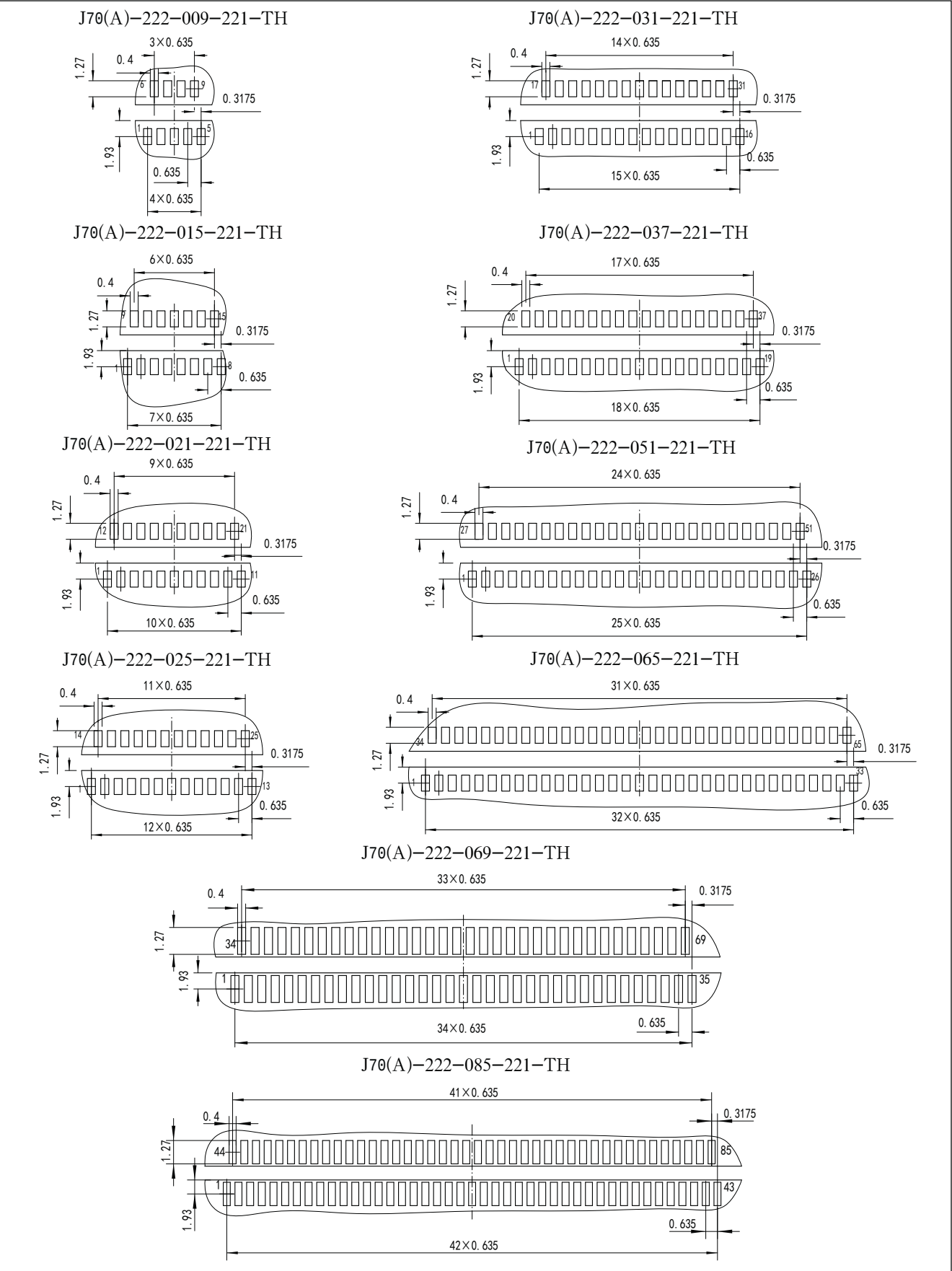
J70(A)-222-XXX-221-TH跨骑表贴（柔性跨接）插座建议焊盘尺寸图
