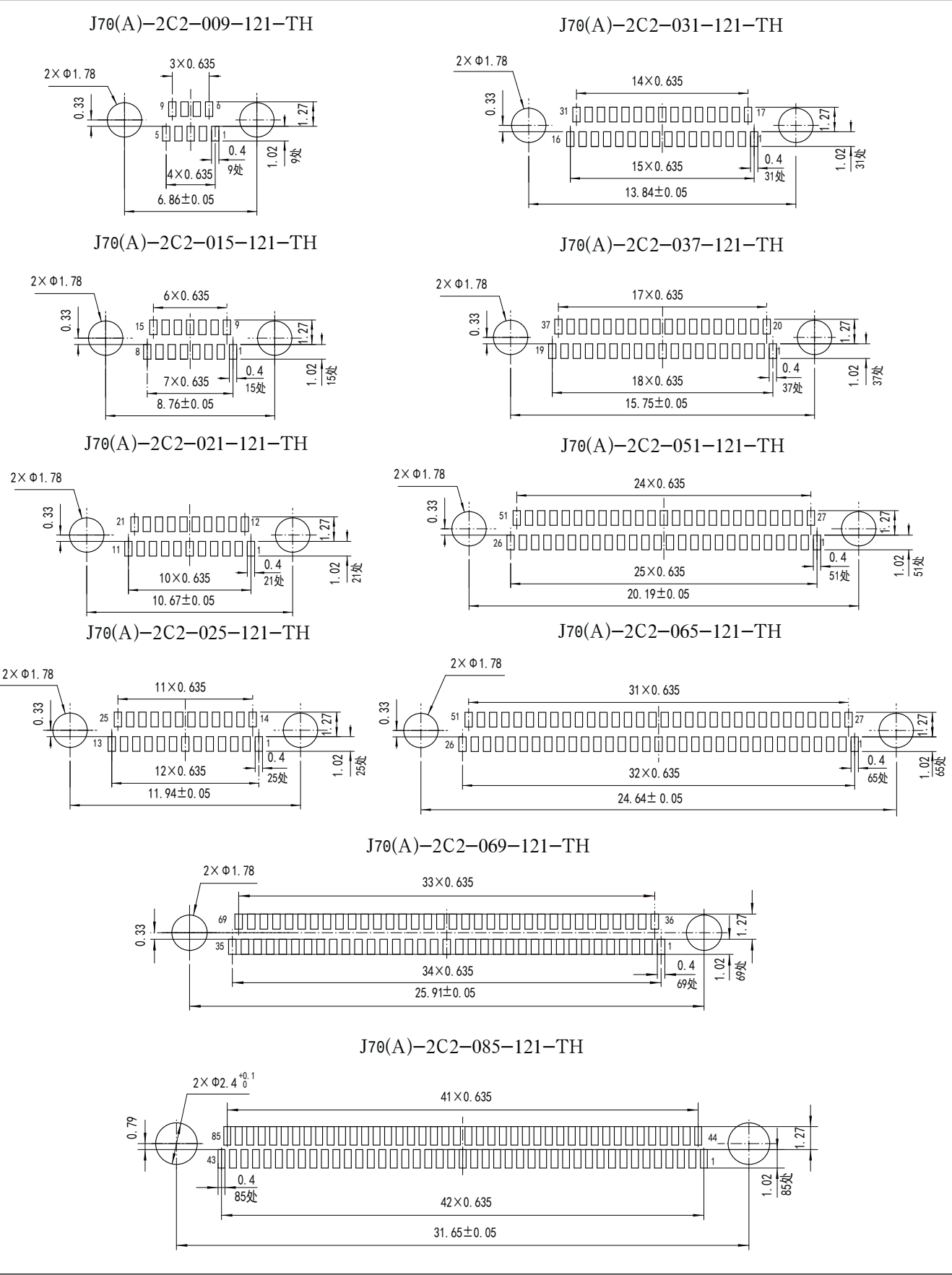
J70(A)-2C2- × × × -121-TH水平表面贴装插头建议印制板开孔及焊盘尺寸图
