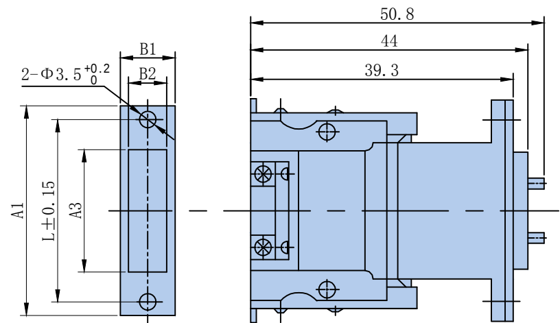
J36A 直插印制板式电连接器外形尺寸结构简图
