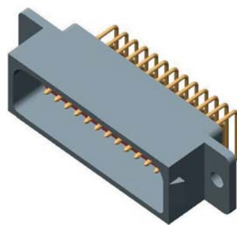
90度弯插印制板插座
