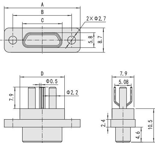
插头J30J□□P□□ □S□□□N3 000 0 产品外形尺寸图
