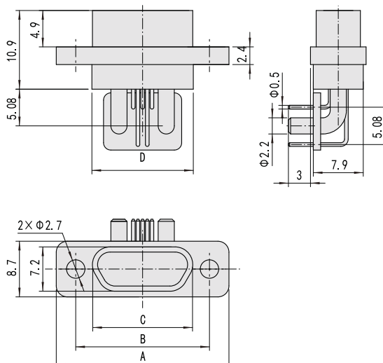
插座J30J□□P□□ □P□□□W1 000 0 产品外形尺寸图
