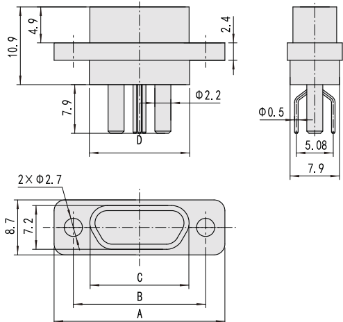
插座J30J□□P□□ □P□□□N3 000 0 产品外形尺寸图
