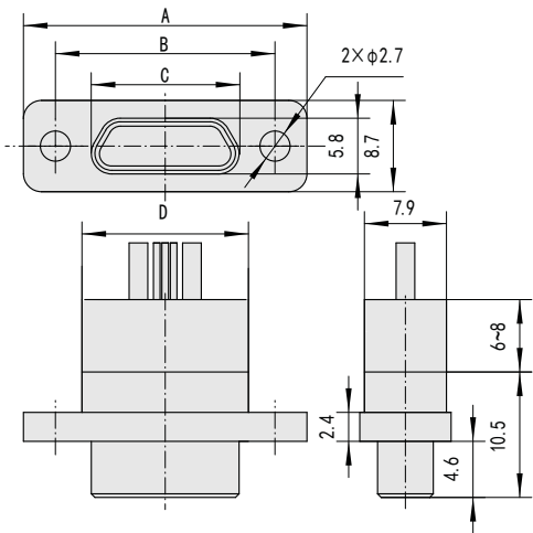
插头J30J□□P□□ □S□□□C0 000 0 产品外形尺寸图
