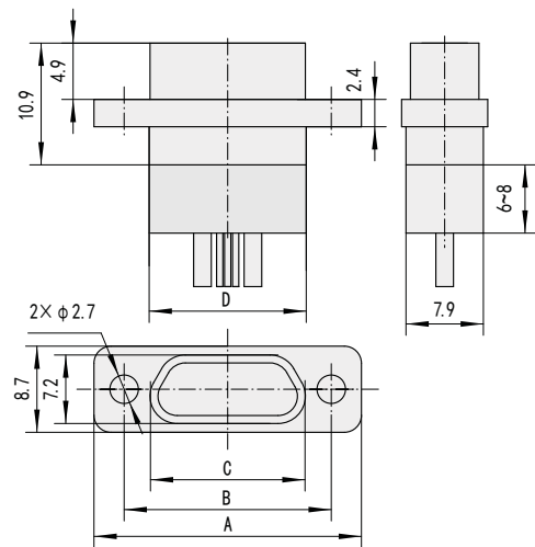
插座J30J□□P□□ □P□□□C0 000 0 产品外形尺寸图
