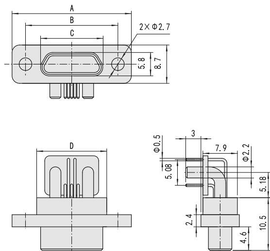
插头J30J□□P□□ □S□□□W1 000 0 产品外形尺寸图
