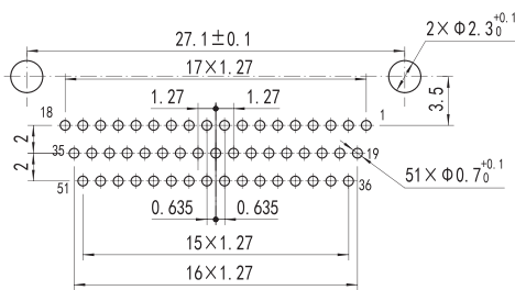
J30JZLN(S) 51ZKWA000
