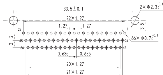
J30JZLN(S) 66ZKWA000
