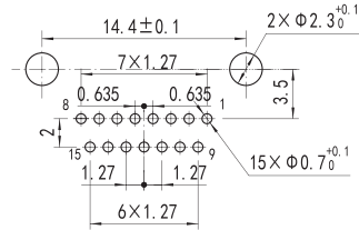
J30JZLN(S) 15ZKWA000
