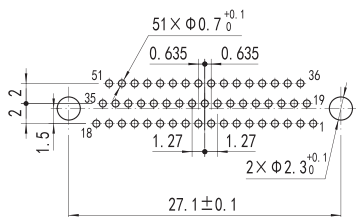
J30JZ/XLN(S) 51TJWA000
