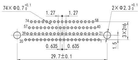
J30JZ/XLN(S) 74TJWA000
