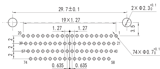
J30JZLN(S) 74ZKWA000
