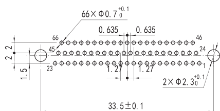
J30JZ/XLN(S) 66TJWA000
