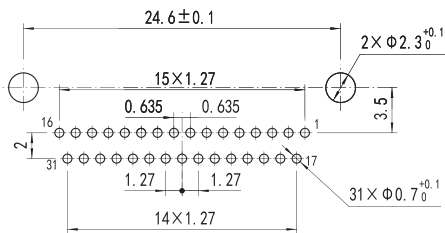
J30JZLN(S) 31ZKWA000
