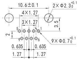
J30JZLN(S) 9ZKWA000
