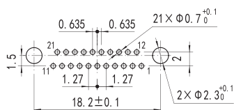
J30JZ/XLN(S) 21TJWA000
