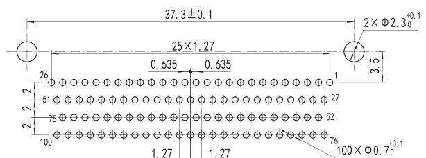
J30JZLN(S) 100ZKWA000
