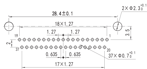
J30JZLN(S) 37ZKWA000
